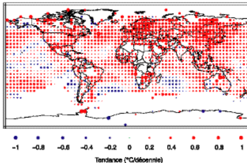
Figure 2: L'hémisphère Nord s'est réchauffé davantage que l'hémisphère Sud. Tendances de la température à la surface du globe, en °C par décennie, calculées à partir des températures annuelles moyennes des années 1976 à 2000. Les tendances sont indiquées par la taille des points (réchauffement en rouge, refroidissement en bleu).
